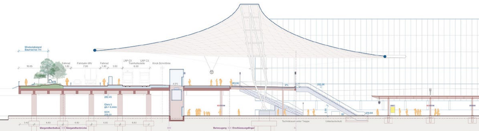
Querschnitt Margarethenbrücke 2035
