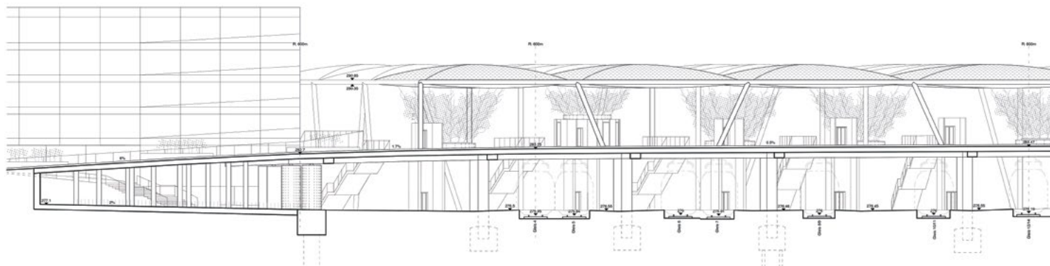
Längsschnitt Margarethenbrücke 2035
