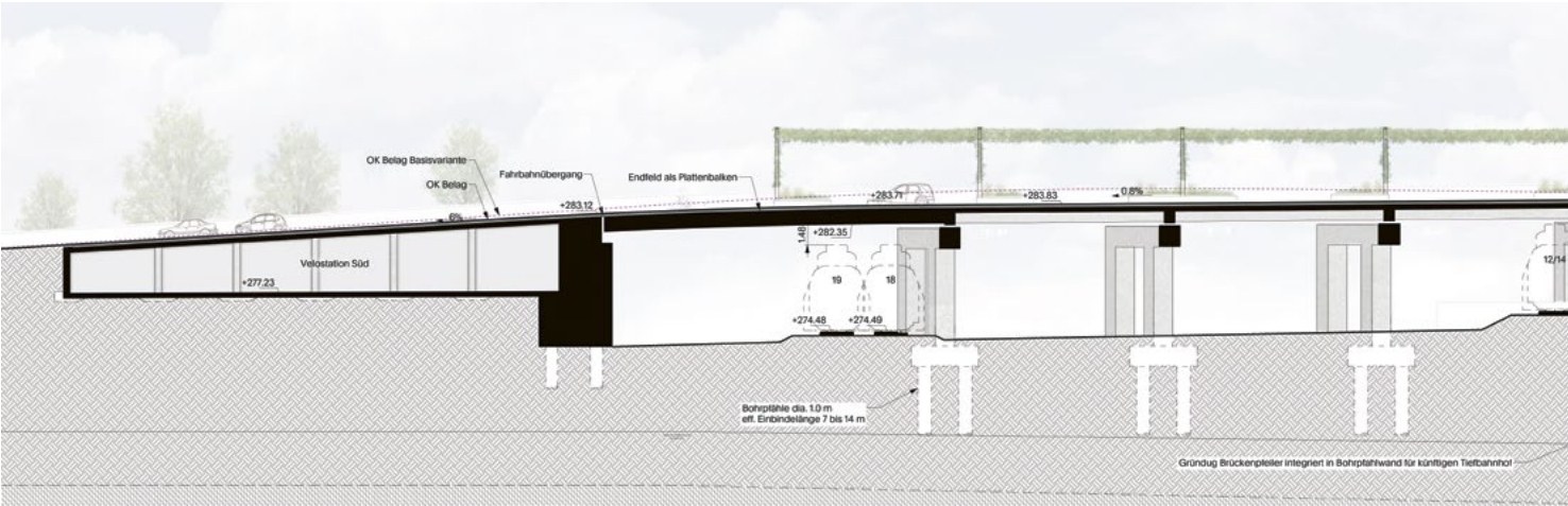
Längsschnitt Margarethenbrücke 2035
