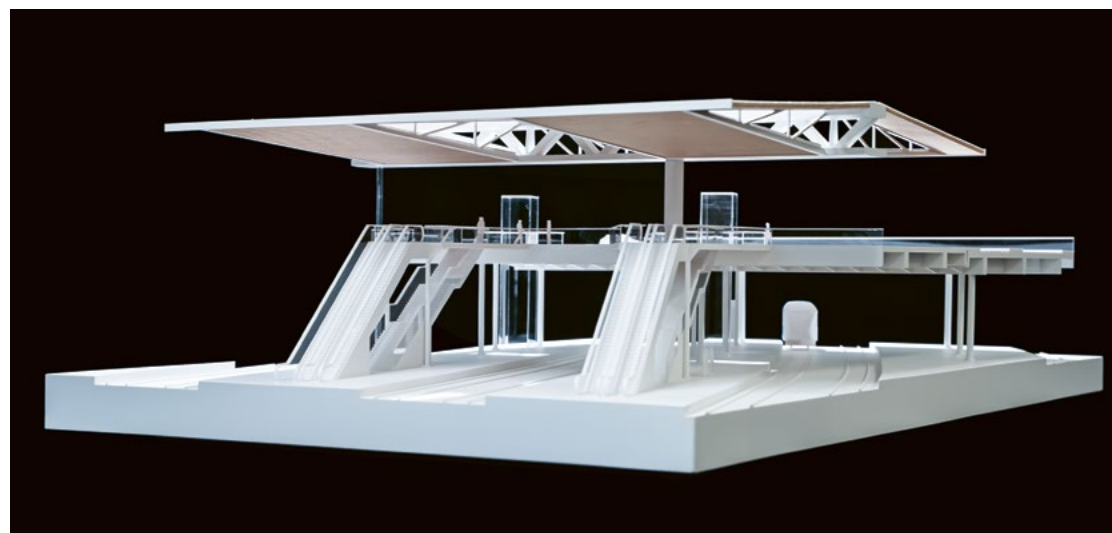
Detailmodell Perronzugang
