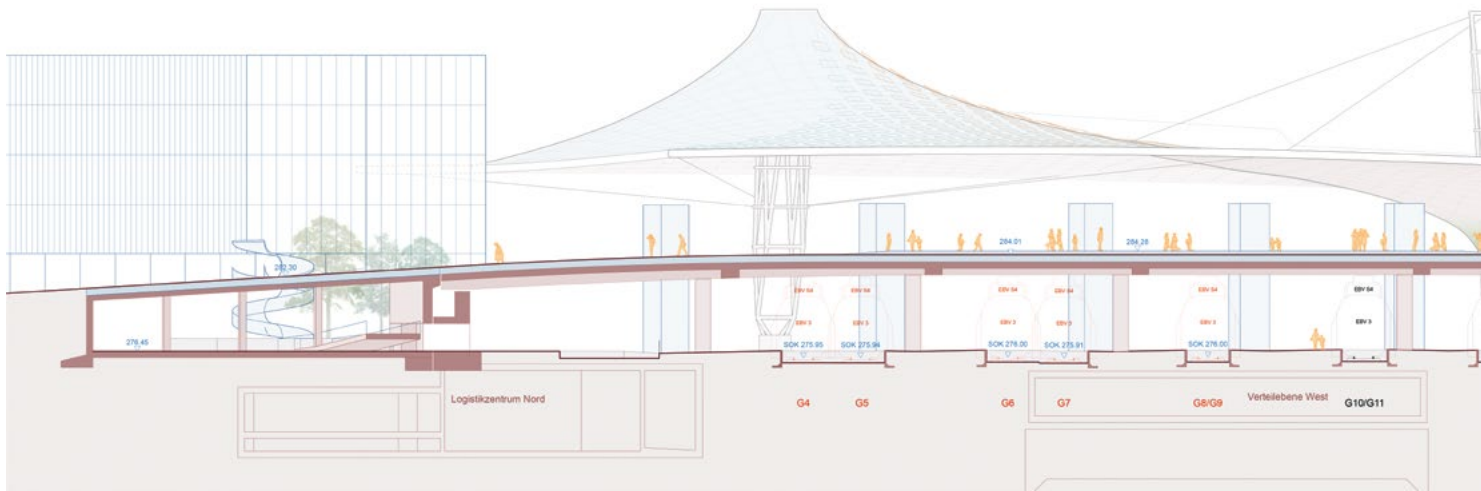
Längsschnitt Margarethenbrücke 2035
