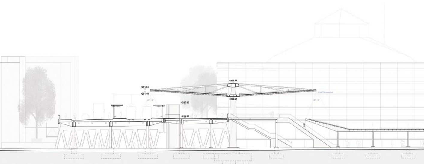
Querschnitt Margarethenbrücke 2035
